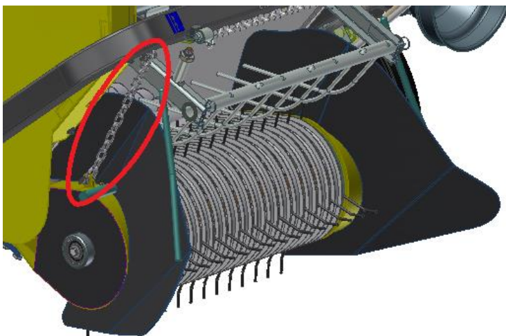
Bild. 25 Einstellkette des Greifers
