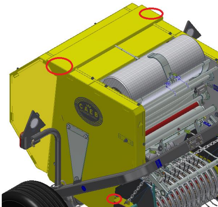
Bild. 41 Schmierungspunkte
