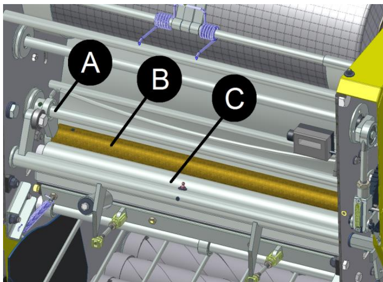
Bild. 37 Antriebsrollen in den Leerlauf versetzen
