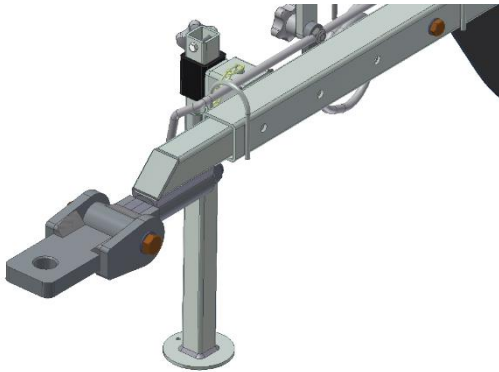
Bild. 8 Tiefliegende, einfache Deichsel
