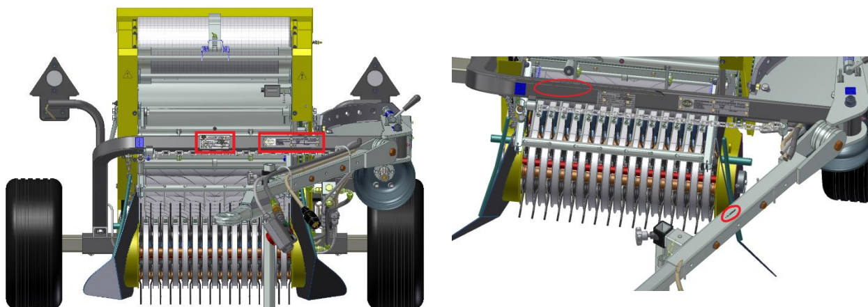
Bild. 3 Position der Schilder und Seriennummer auf dem Fahrgestell
