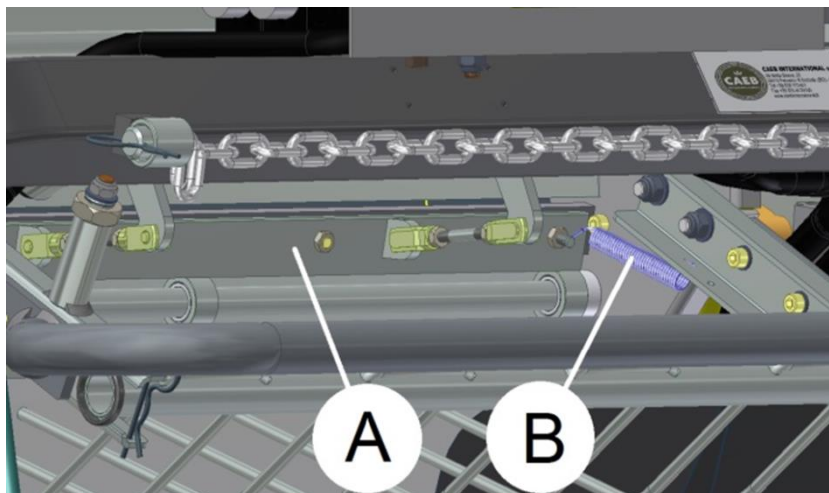
Bild. 33 Rückstellfedern des Kontermessers
