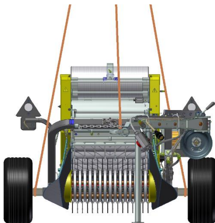
Bild. 16 Verseilung für Hebung
