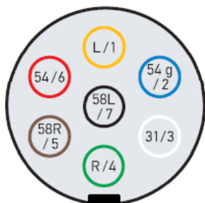
Bild. 50 Anordnung der Steckdosenkontakte Typ 12N
