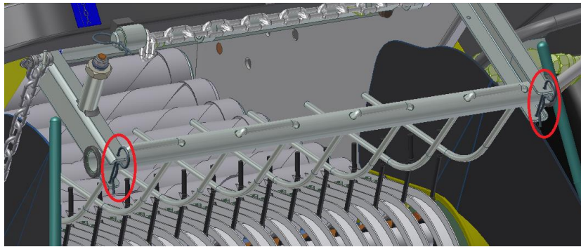
Bild. 34 Position der elastischen Splints des Förderrechen
