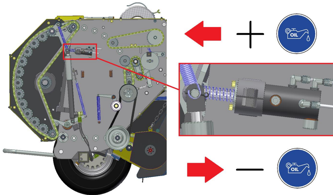
Bild. 31 Einstellung der Schmierpumpe
