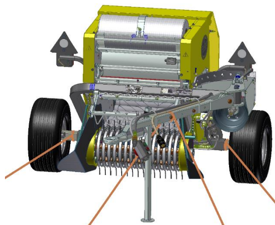
Bild. 17 Verankerung
