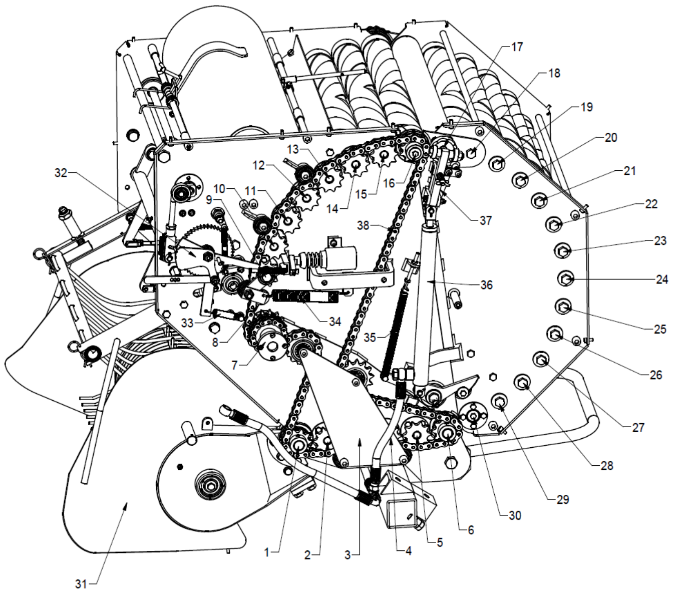
Bild. 48 Ziffern für die Feststellung der Übergruppen an der linken Seite (Fahrrichtung)
