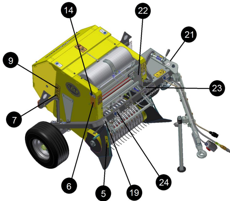
Bild. 14 Position der nummerierten Piktogramme aus der linken Vorderansicht
