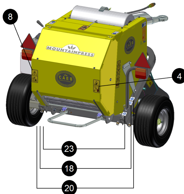
Bild. 15 Position der nummerierten Piktogramme aus der linken Hinteransicht
