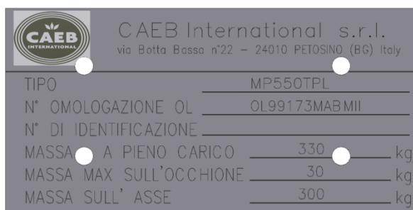
Bild. 2 Schild mit Serien- und Zulassungsnummer
