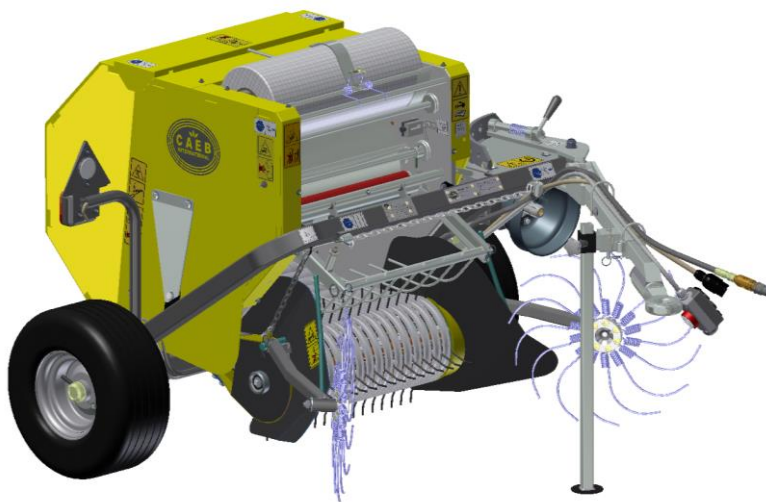
Bild. 10 Schwadenräder
