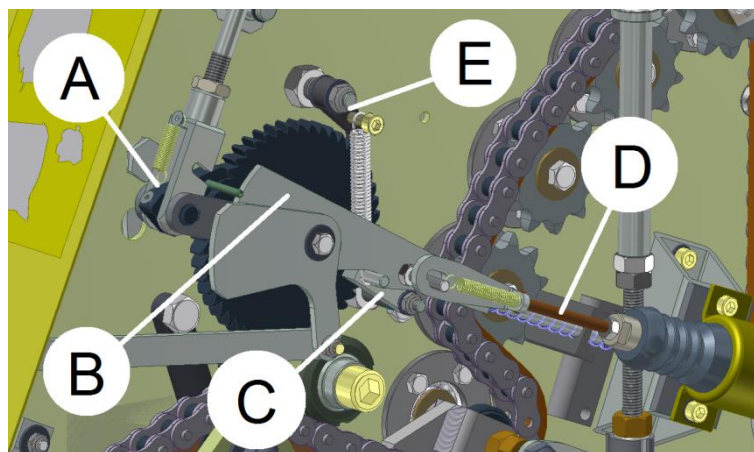
Bild. 44 Reinigung des Bindungsmechanismus
