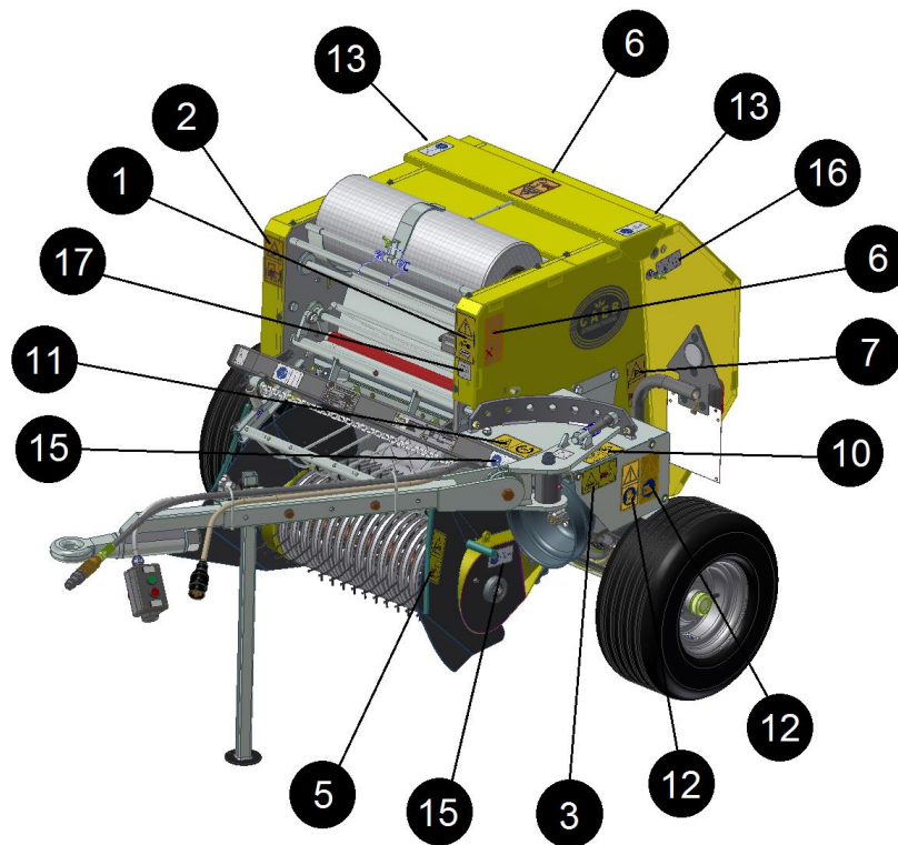
Bild. 13 Position der nummerierten Piktogramme aus der rechten Hinteransicht
