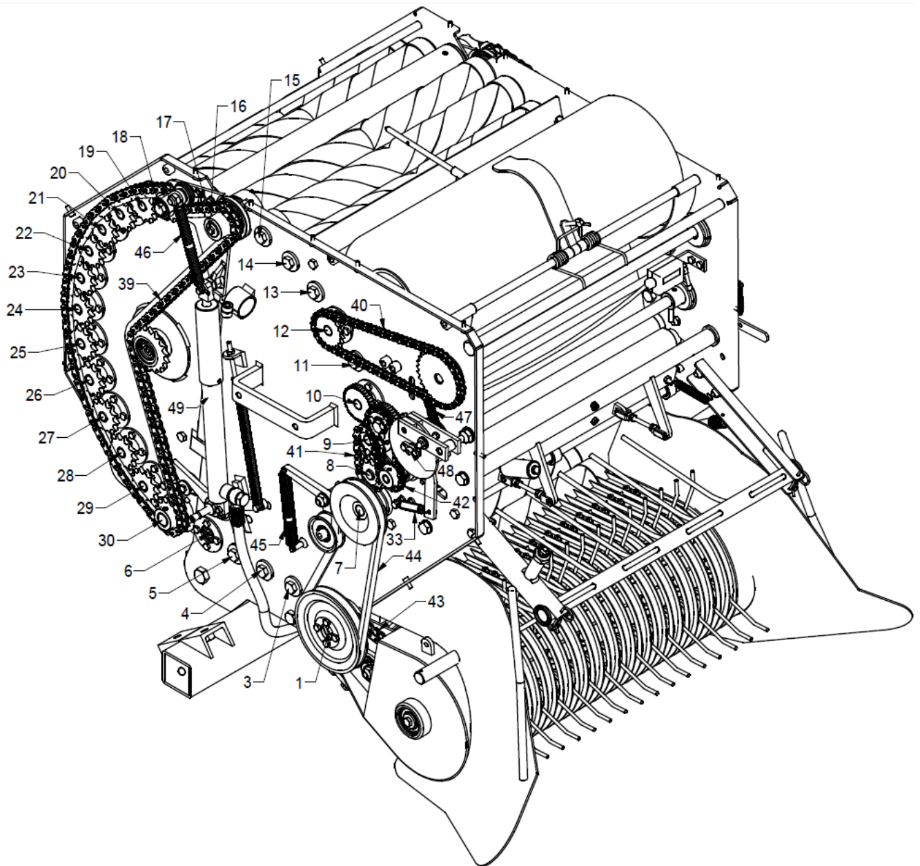
Bild. 49 Ziffern für die Feststellung der Übergruppen an der rechten Seite (Fahrriichtung)
