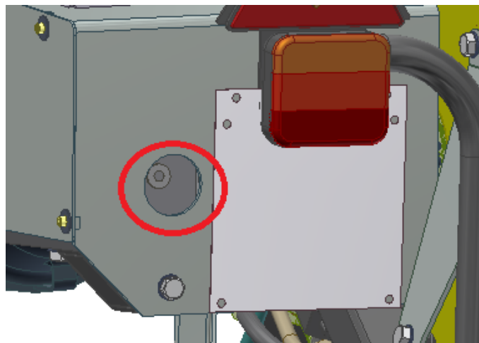
Bild. 42 Einfüllstopfen für Winkeltrieböl
