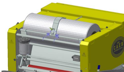
Bild. 7 Schmierung
