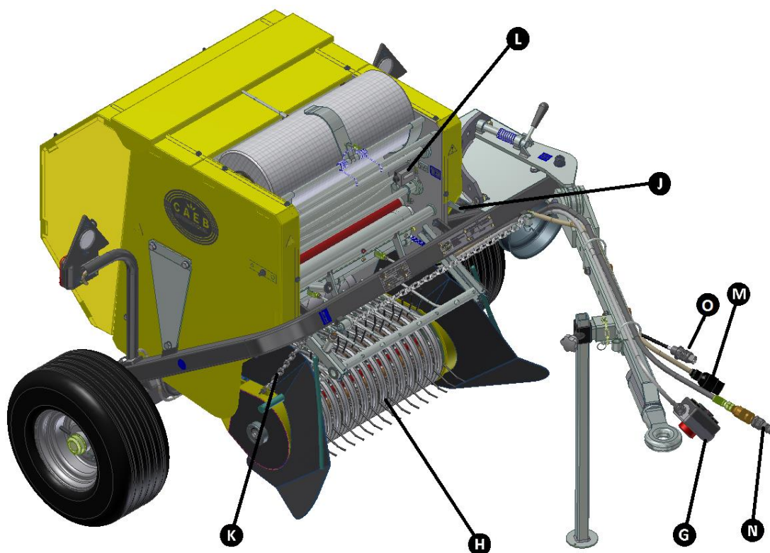
Bild. 5 Bauteile der Maschine
