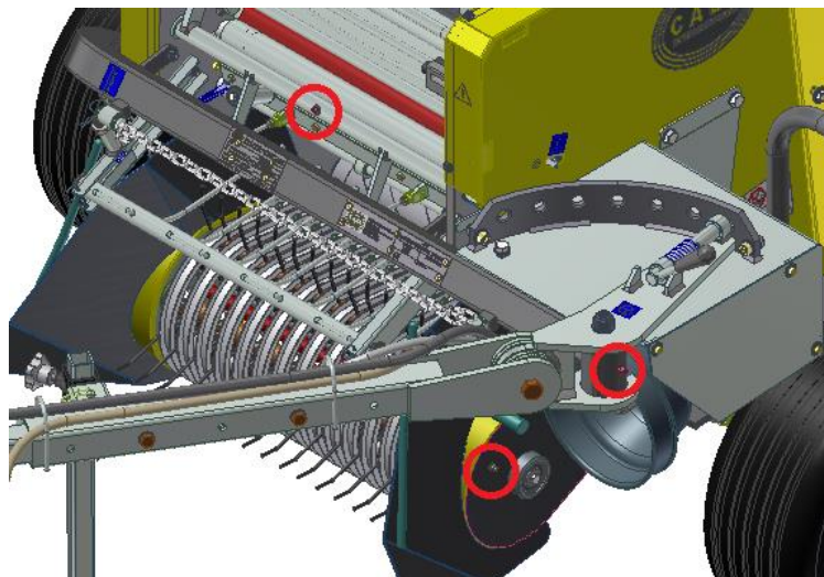
Bild. 40 Einfettungspunkte
