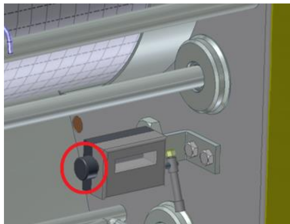
Bild. 29 Position des Rundballenzählers und Rücksetzrädchen
