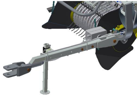
Bild. 9 Tiefliegende, doppelte Deichsel
