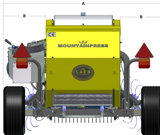
Bild. 24 Fahrspurbreite
