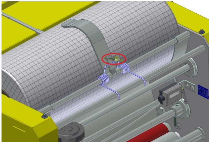
Bild. 32 Einstellung der Netzbremse
