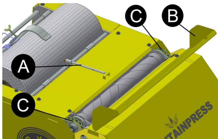
Bild. 39 Schmierpunkte der Rollenantriebsketten
