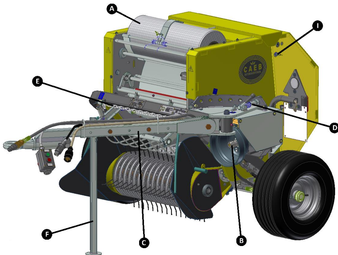
Bild. 4 Bauteile der Maschine
