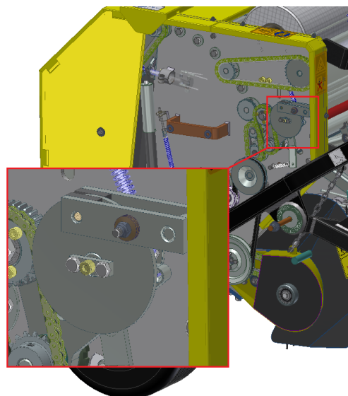
Bild. 36 Freno legatura Bindungsbremse
