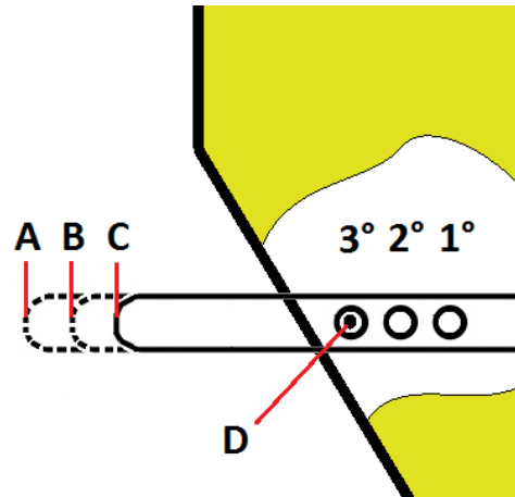
Bild. 28 Positionen des Einstellhebels für Netzumwicklungen
