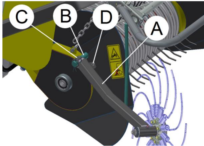
Bild. 30 Montage der Schwadenräder
